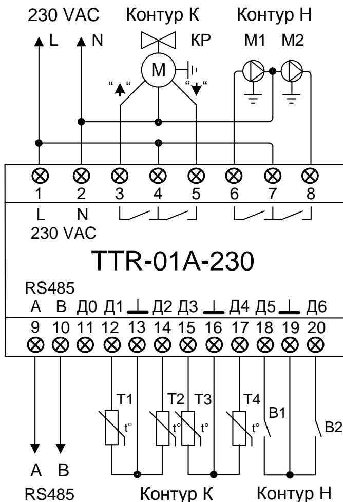
Рисунок В.1 - Схема электрическая подключений TTR-01A-230
