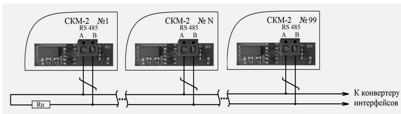
Рисунок Г.7 – Схема организации сети счетчиков на базе интерфейса RS485
