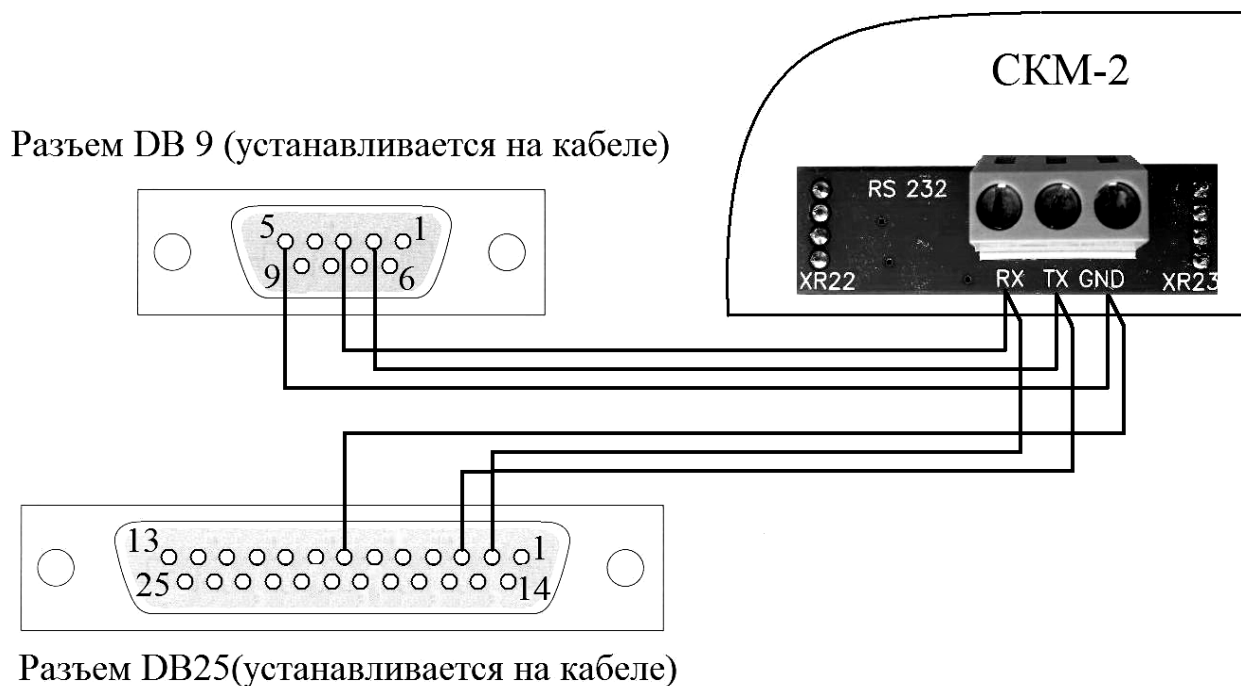
Рисунок Г.6 – Схема подключения счетчика к модему
