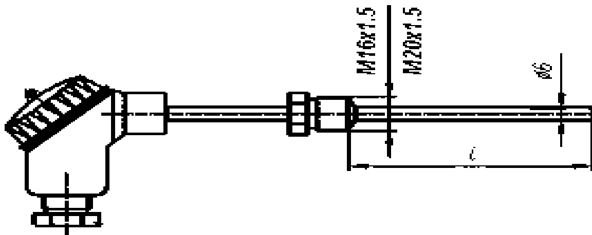
Рисунок Е.5 – Термопреобразователь
