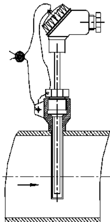
Рисунок Е.3 – Схема монтажа термопреобразователя без защитной гильзы на трубопроводе
