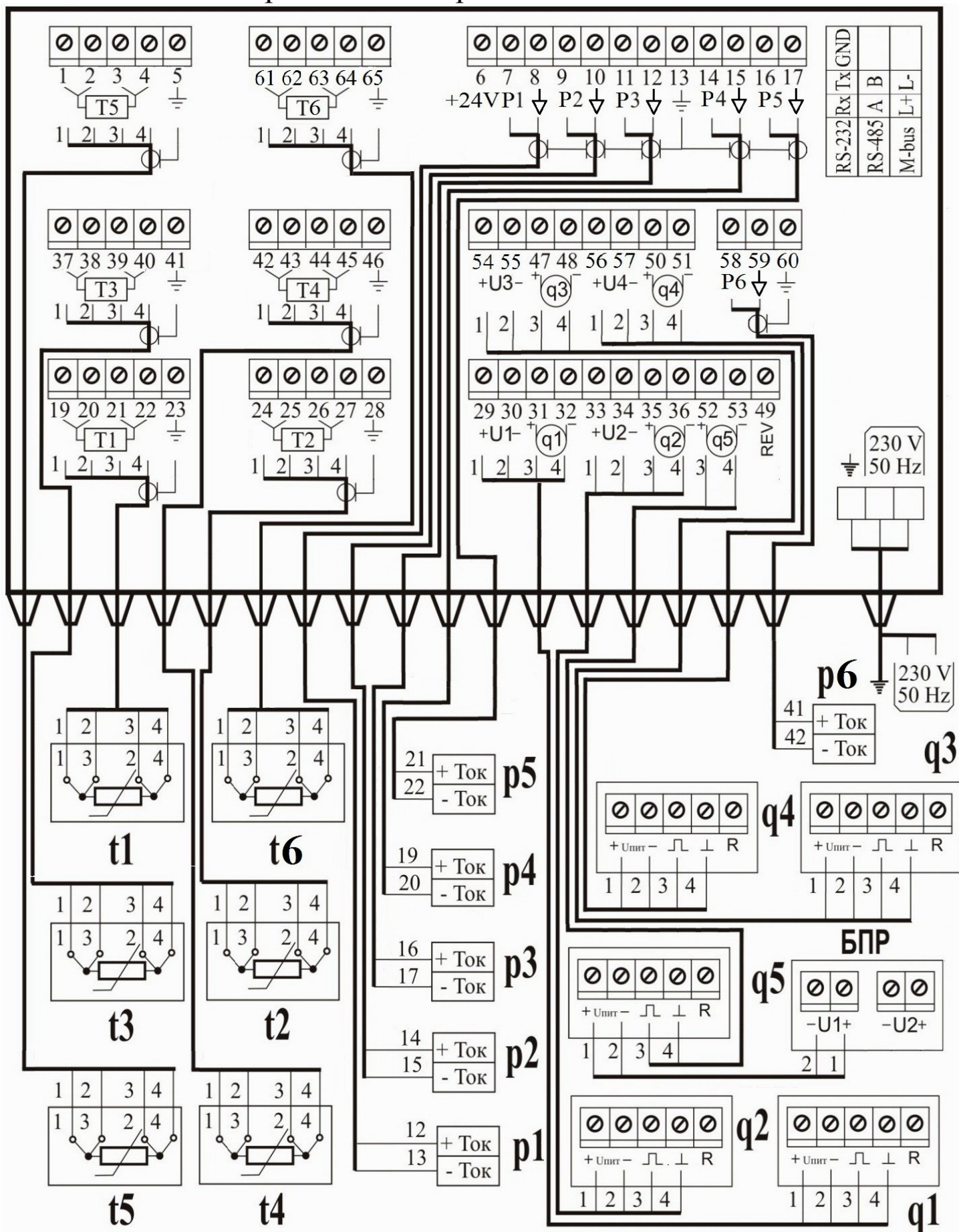
Рисунок Г.2 – Схема электрическая подключения вычислителя СКМ-2 МНОГОКАНАЛЬНОГО
