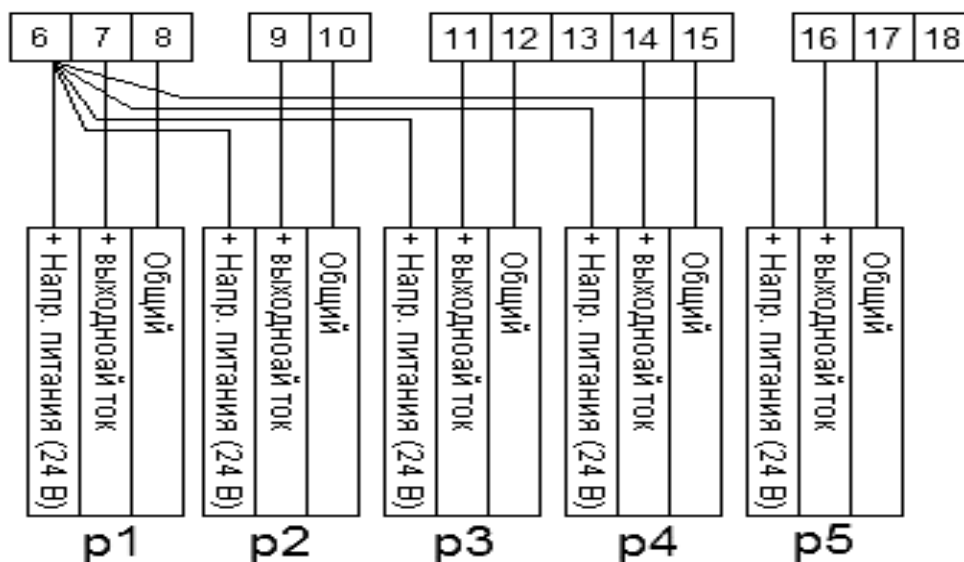
Рисунок Г.3 – Трехпроводная схема подключения преобразователей давления, питание от вычислителя +24 В
