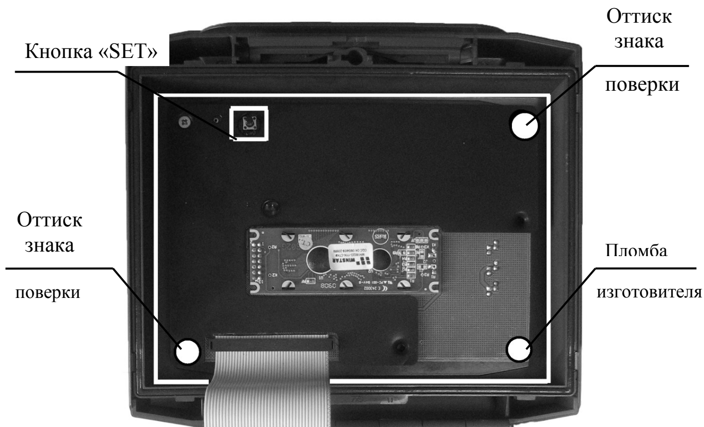
Рисунок Е.2 – Вид вычислителя с открытой крышкой (корпус Vorla)
