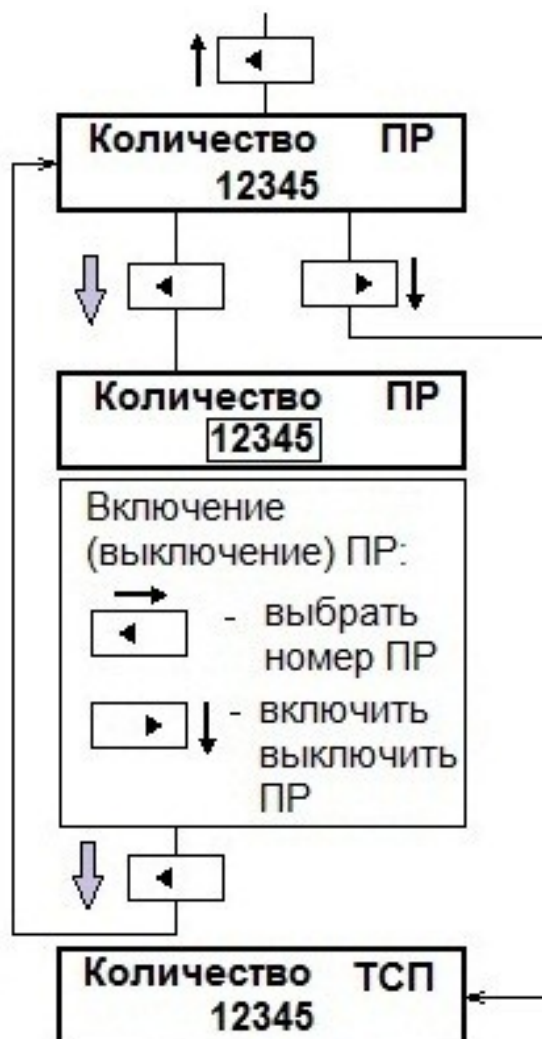
Рисунок 12 – Схема ввода настроечных параметров №4
