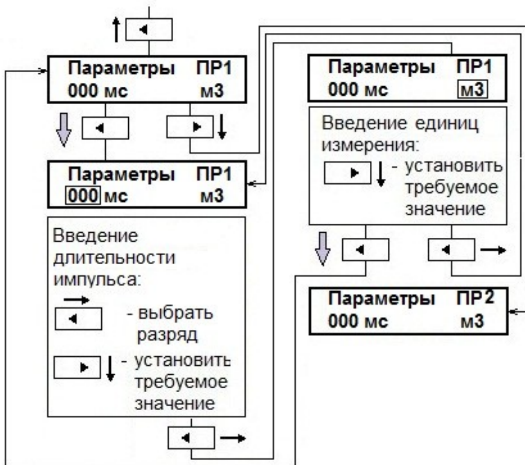
Рисунок 13 – Схема ввода настроечных параметров №5
