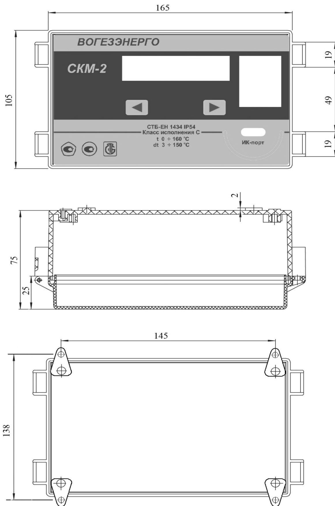
Рисунок В.1 – Габаритные и установочные размеры вычислителя двухканального (корпус Sanhe)
