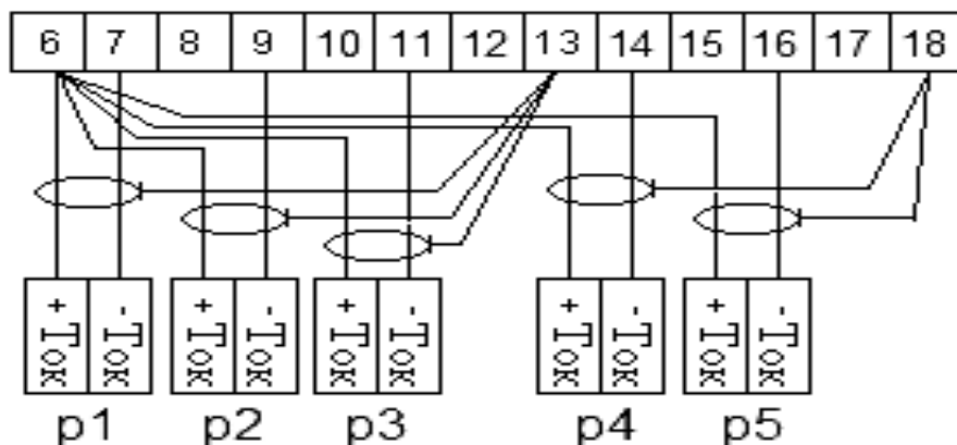
Рисунок Г.2 – Двухпроводная схема подключения преобразователей давления (4-20 мА), питание от вычислителя +24 В
