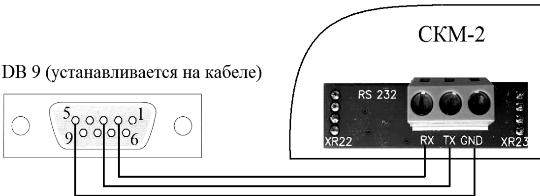
Рисунок Г.5 – Схема подключения счетчика к компьютеру
