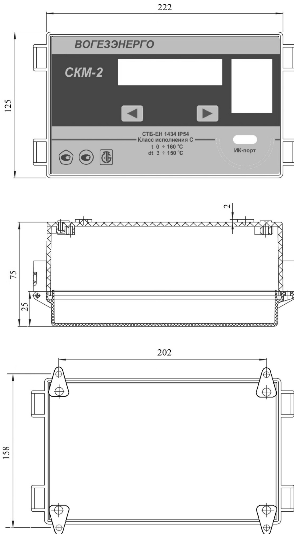
Рисунок В.3 – Габаритные и установочные размеры вычислителя многоканального (корпус Sanhe)
