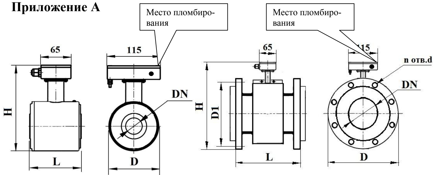
а) исполнение «сэндвич» серии 1000, 2000.
